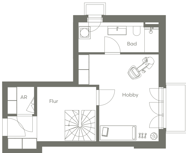
UNTERGESCHOSS
