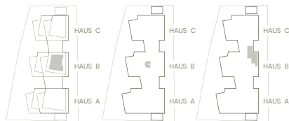
DACHAUFSICHT / DACHGESCHOSS
